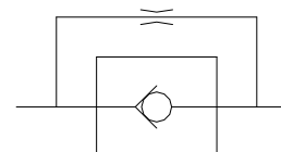
ANSI SYMBOL
